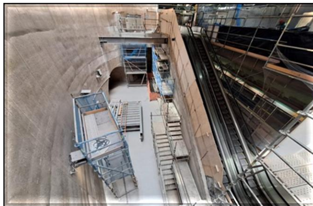
Linha 2-Verde - Plataforma 2 - lado leste: novas escadas, fixa e rolante, inauguradas em 23/12/2024.
