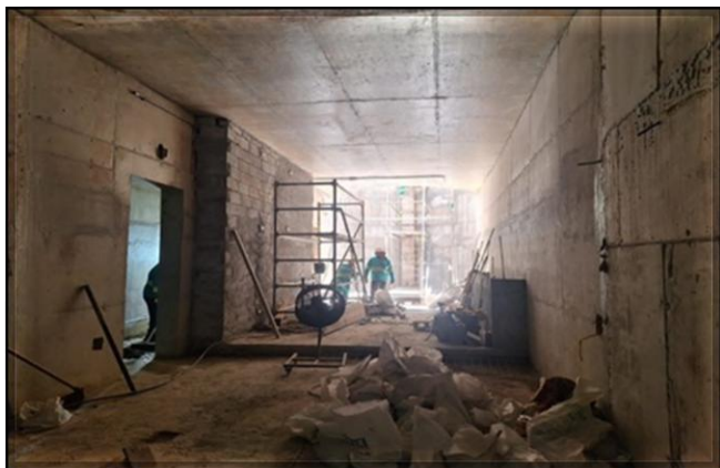
Exaustão 1 - Novo canal de ventilação da Plataforma 2 da estação Vila Prudente da Linha 2-Verde: montagem e testes do sistema de ventilação.
