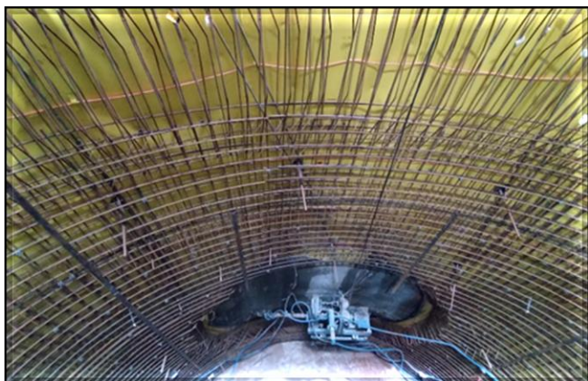
Poço principal: armação concluída e vista do emboque do túnel sul (sentido Estação Paulista)
