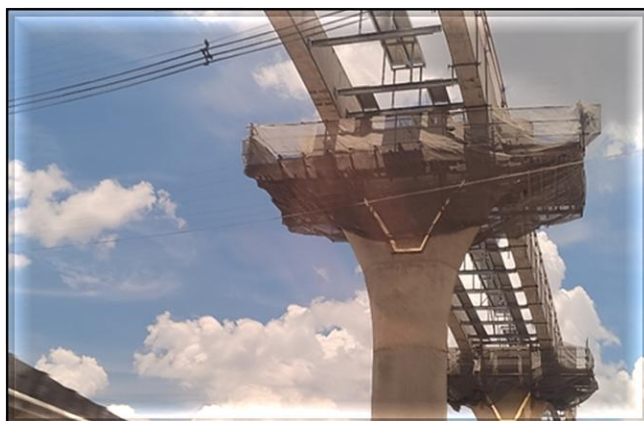
Obra Civil – instalação da passarela de emergência.
