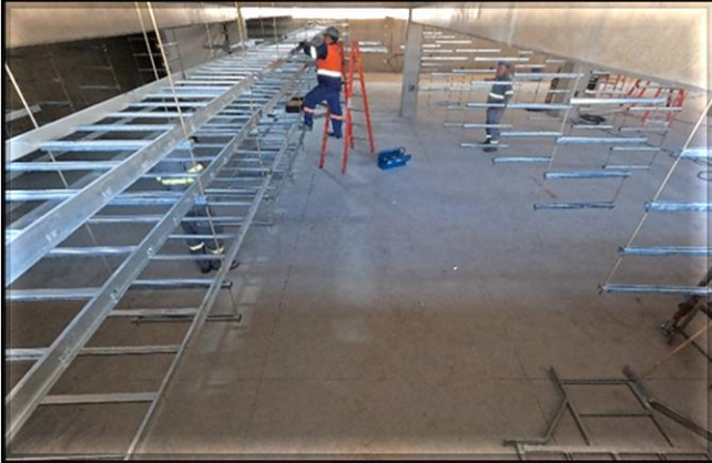
Instalação do bandejamento em execução nos porões de cabos do Edifício de Salas Técnicas.
