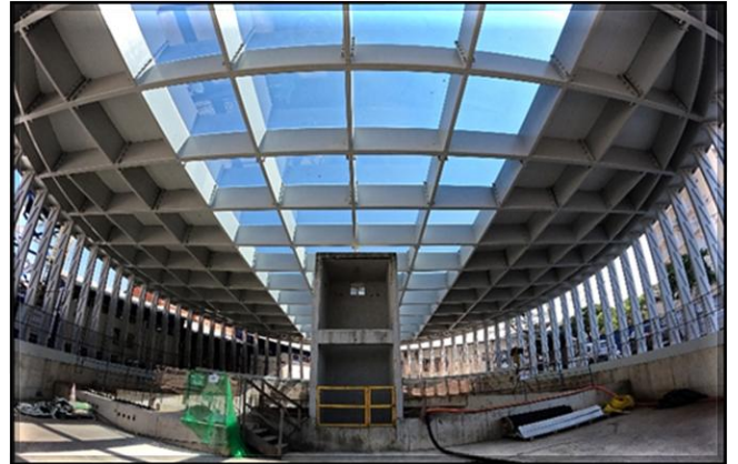
Vidros instalados na cobertura metálica do Acesso A.
