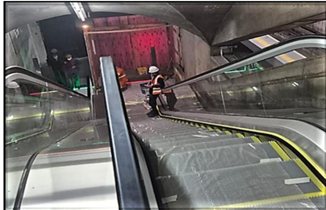
Escada Rolante (ER 25 – lado oeste) – Montagem Concluída
