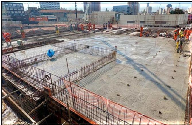
Concretagem das lajes das salas técnicas em execução.
