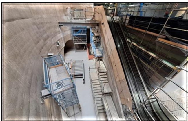
Linha 2-Verde - Plataforma 2 - lado leste: montagem da nova escada fixa.
