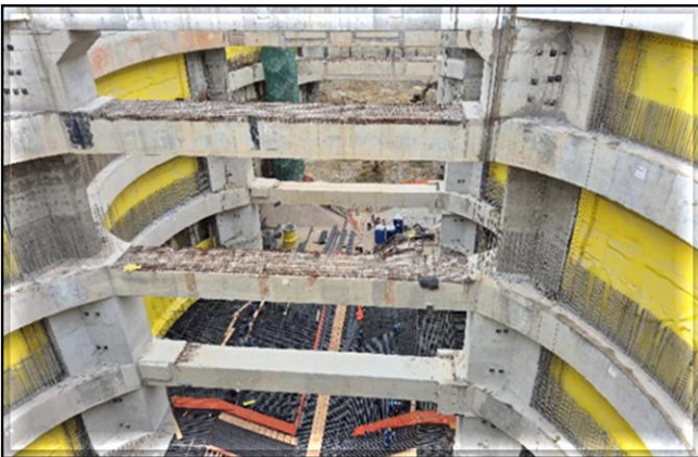
Início da concretagem da laje de fundo do corpo da estação.
