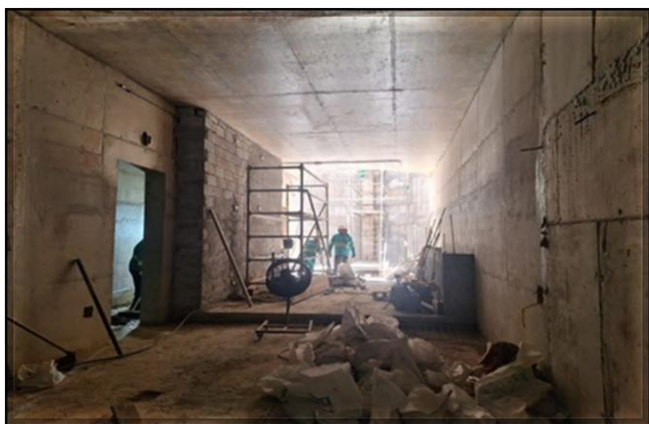
Exaustão 1 - Novo canal de ventilação da Plataforma 2 da estação Vila Prudente da Linha 2-Verde: concretagem concluída, em andamento o acabamento e a preparação do piso.
