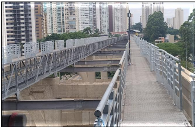
Vias do Monotrilho/Civil – instalação dos guarda-corpos na passarela de emergência.
