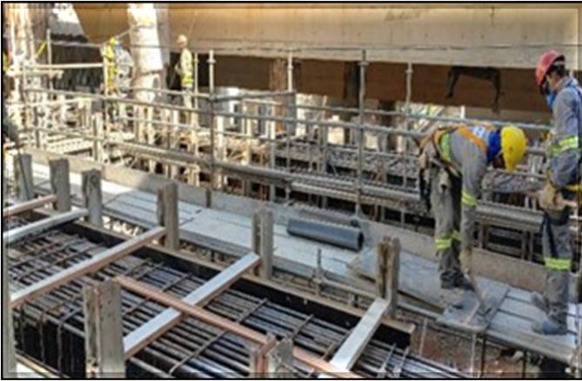
Estruturas de concreto e escavação do corpo da estação.
