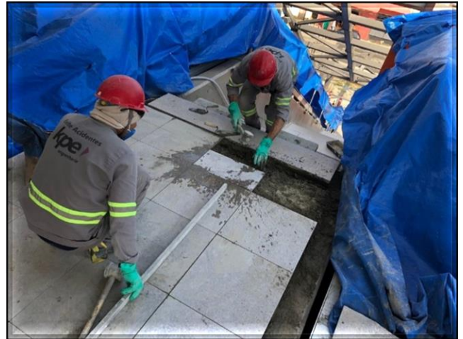
Acesso A – Obra civil – execução do piso de granito.
