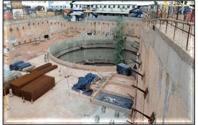
Escavação do poço do corpo da estação.
