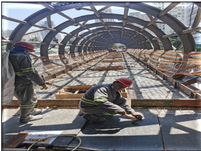
Passarela – Obra Civil – execução de caixa de passagem para a concretagem do contrapiso
