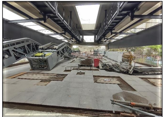
Mezanino – Obra civil – execução do piso de granito. Sistemas – escada rolante a ser posicionada.
