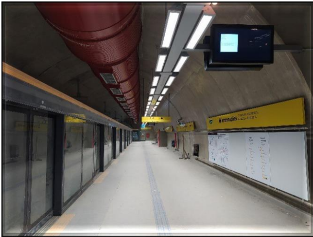
Corpo da Estação – Sistemas de Telecomunicações e Portas de Plataformas comissionados..
