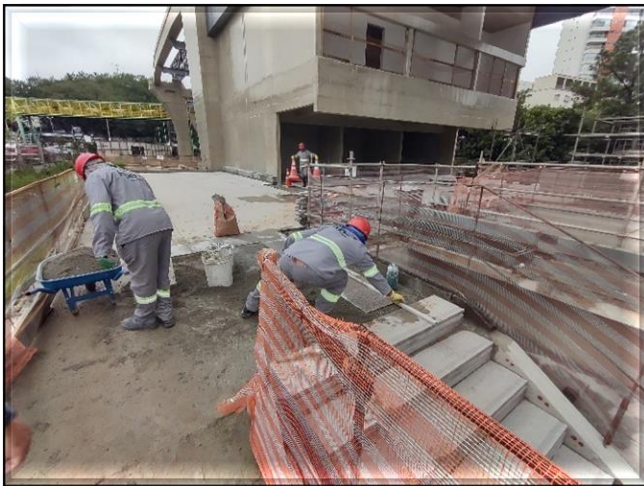
Acesso - execução do piso de granito.
