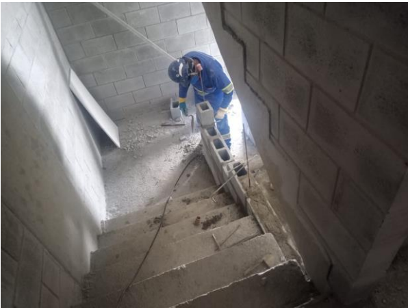
Obra Civil – execução de alvenaria das escadas do ETO.
