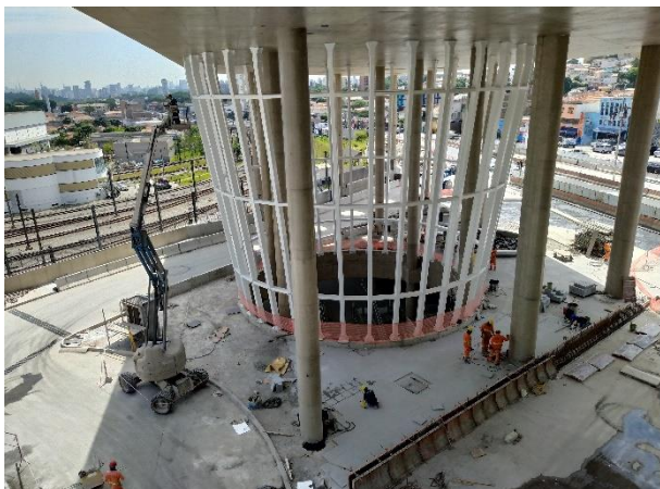
Acesso Heitor dos Prazeres – execução da estrutura metálica do cone de vidro.
